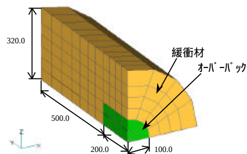
図-1 解析モデル (単位 mm)
