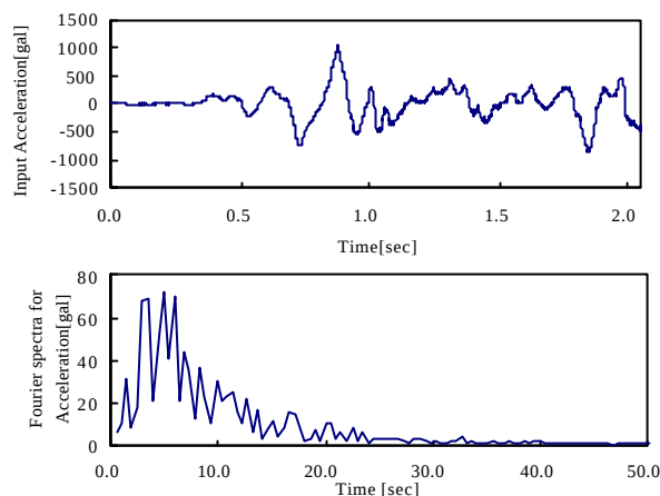
図-2 入力地震動 (Imperial Valley)
