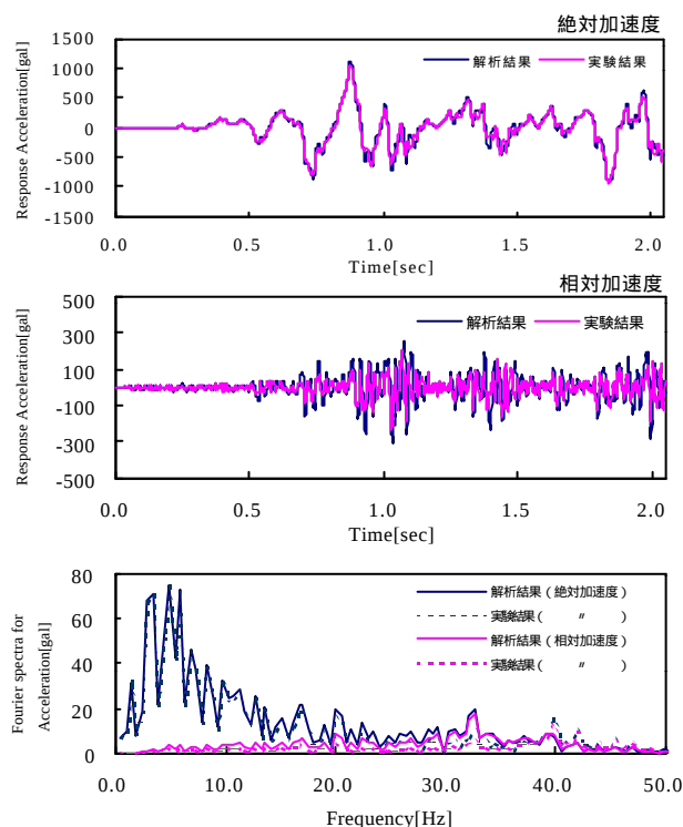
図-3 応答加速度の比較
