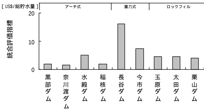
図-2 貯水量あたりの環境負荷の統合評価
