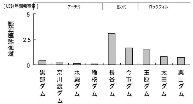
図-3 年間発電量あたりの環境負荷の統合評価
