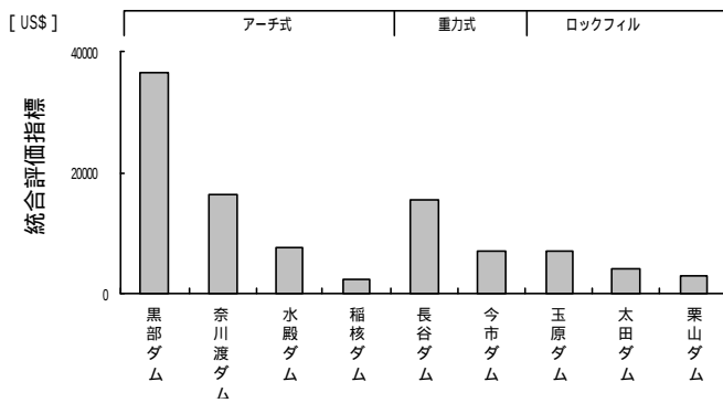
図-1 ダム構造物における環境負荷の統合評価
