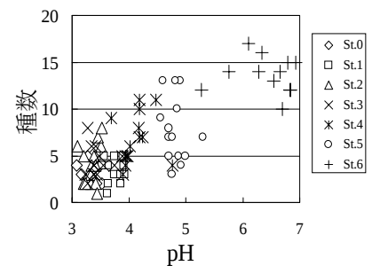
図-4 pH と種数
