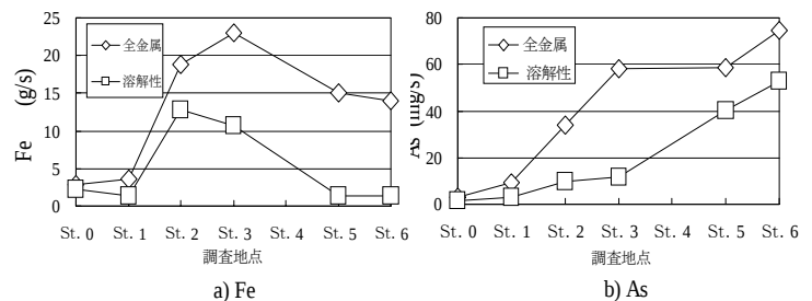
図-3 流下方向における負荷量の変化('99.10.)
