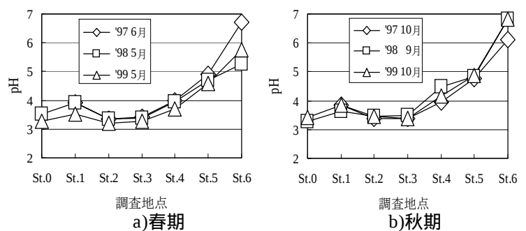
図-2 流下方向におけるpHの変化
