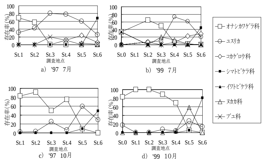
図-5 流下方向における存在率の変化
