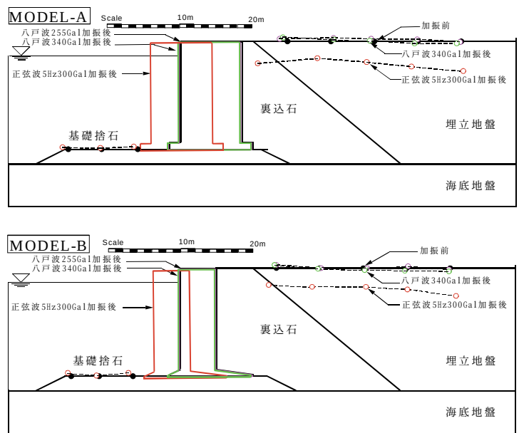
図-3 変形状態図
