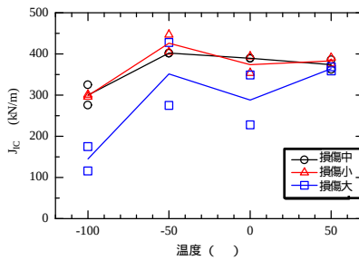
図 6 SP 試験における J_{IC} 値と温度の関係
