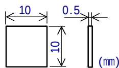
図 1 SP 試験片形状
