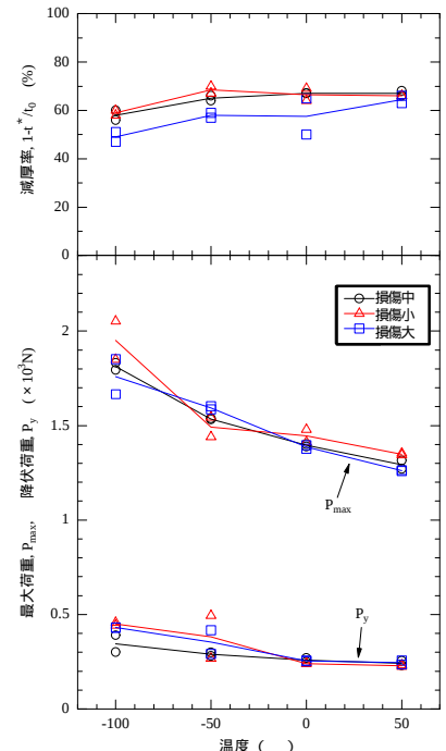
図 7 SP 試験における最大荷重、降伏荷重、減厚率と温度の関係
