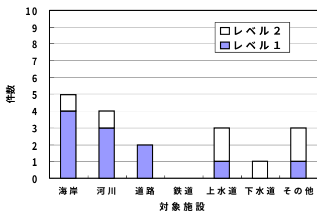
図-2 対象構造物の施設別件数（地震力区分）
