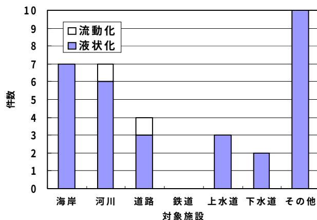
図-3 対象構造物の施設別件数(液状化・流動化区分)
