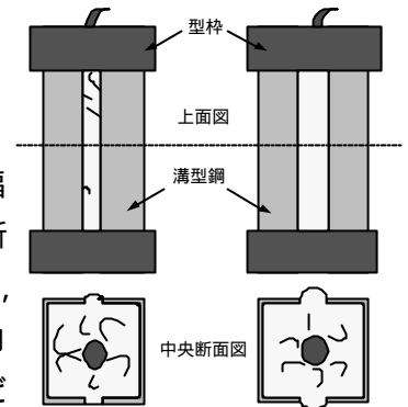
図-3 隙間の袋形状概略図
