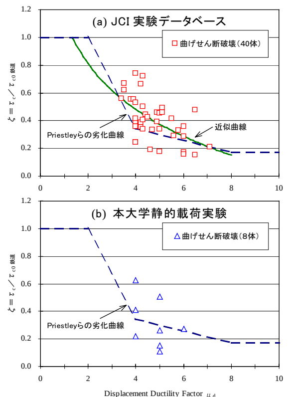
図-1 実験終局時のせん断強度劣化 \zeta
