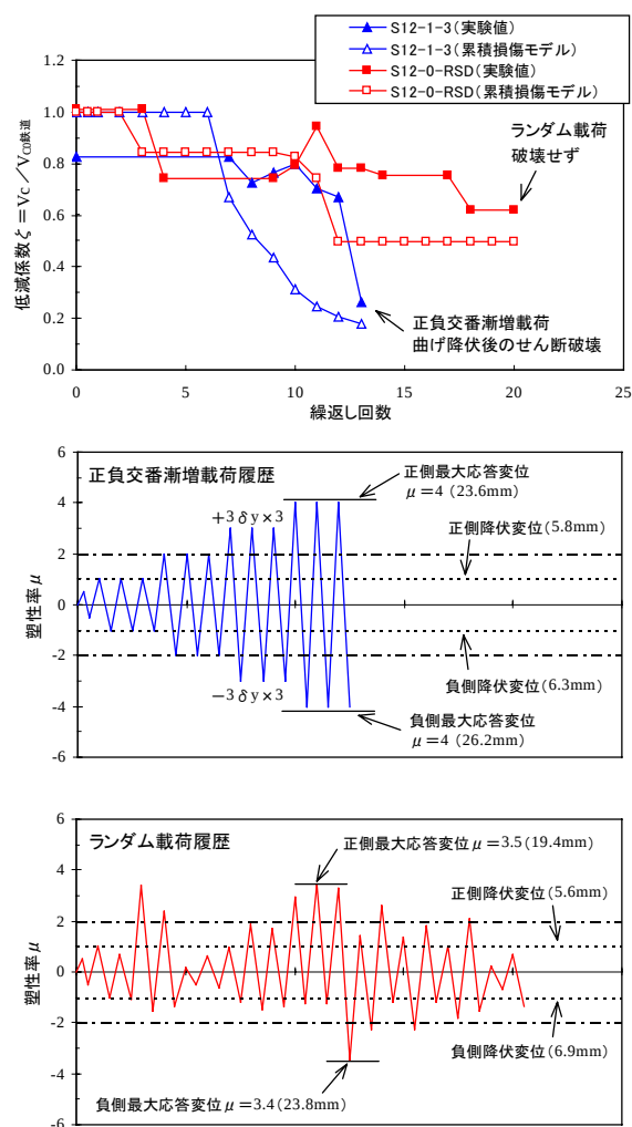
図-2 サイクル上のせん断劣化過程
