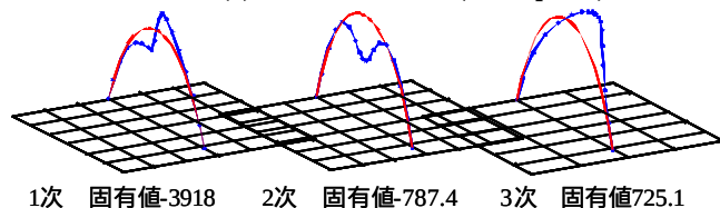
図 - 2 (b) 固有モード (bifurcation point)
