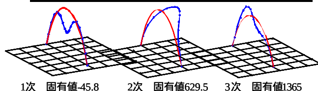
図 - 2 (a) 固有モード (limit point)
