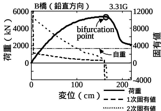
図 - 1 荷重 - 変位曲線と固有値の変化 (B 橋)
