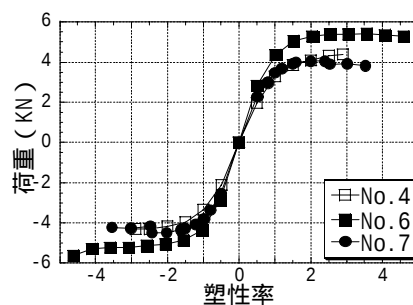
図 - 3 荷重—塑性率 (RC)
