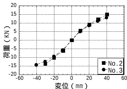
図 - 2 荷重—変位 (Steel)
