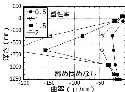
図 - 4 深さ—曲率 (No. 4)
