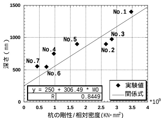
図 - 6 曲率最大点深さ - 杭、地盤の相対剛性関係
