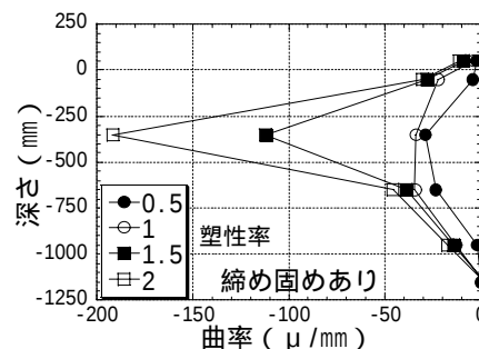
図 - 5 深さ—曲率 (No. 6)
