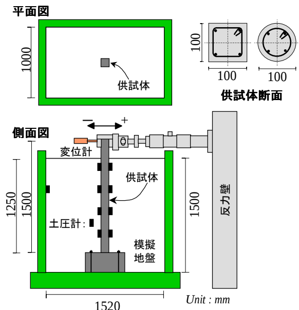
図 - 1 実験概要図
