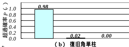
図6 対象橋脚の耐震性能評価
