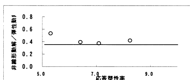
図 4 応答塑性率と非線形動解結果/弾性動解結果関係 (応答変位)
