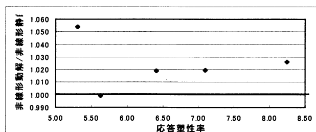
図 6 応答塑性率と非線形静的結果/非線形動解結果関係 (応答せん断力)
