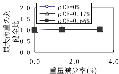
図3 重量減少率が最大荷重に与える影響
