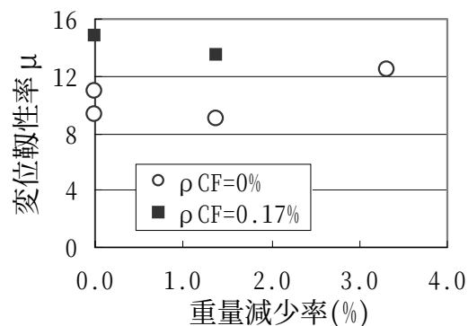
図4 重量減少率が変位靱性率に与える影響
