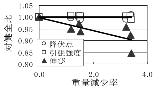
図2 重量減少率が鉄筋の機械的性質に与える影響
