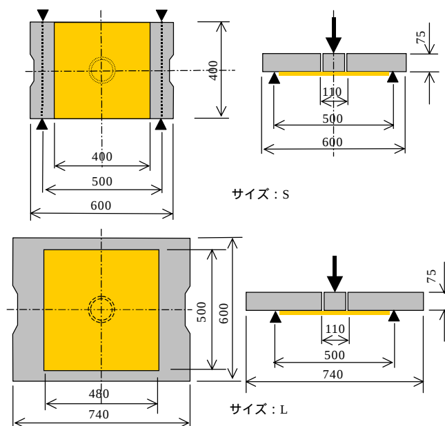
図 - 1 押し抜き試験体
