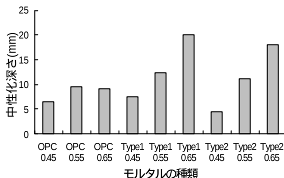
図 2 各種モルタルの中性化深さ
