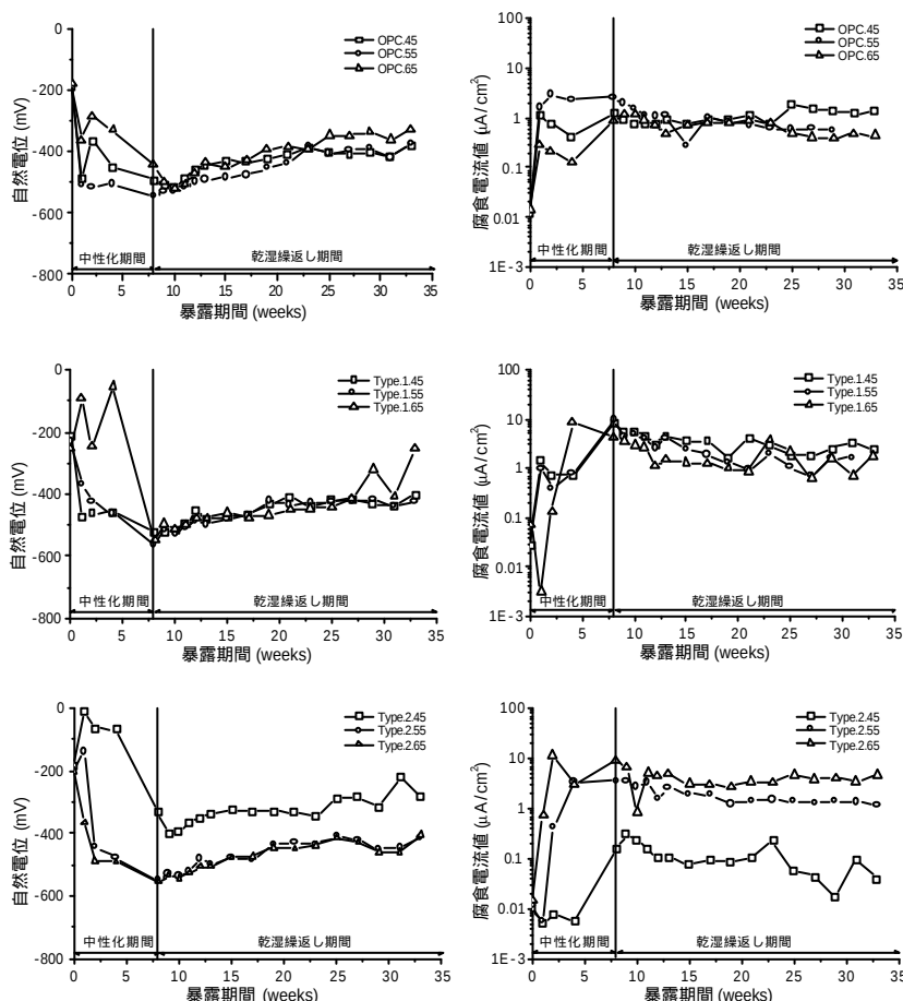
図 3 自然電位の経時変化
