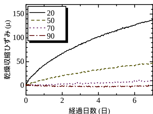
図 - 4 W/B が 25 % の場合の乾燥収縮ひずみ
