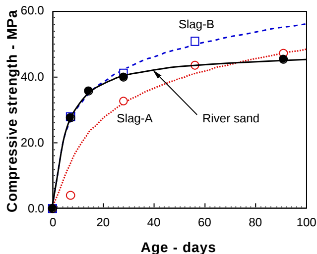
図2 銅スラグを用いたコンクリートの強度
