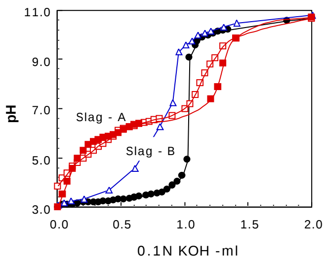
図3 酸・塩基適定試験の適用
