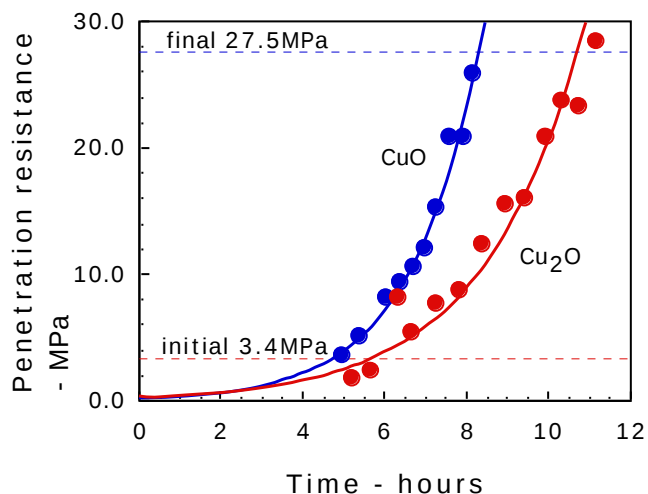
図5 酸化銅による凝結遅延効果
