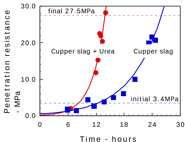
図6 尿素の添加による凝結遅延抑制効果
