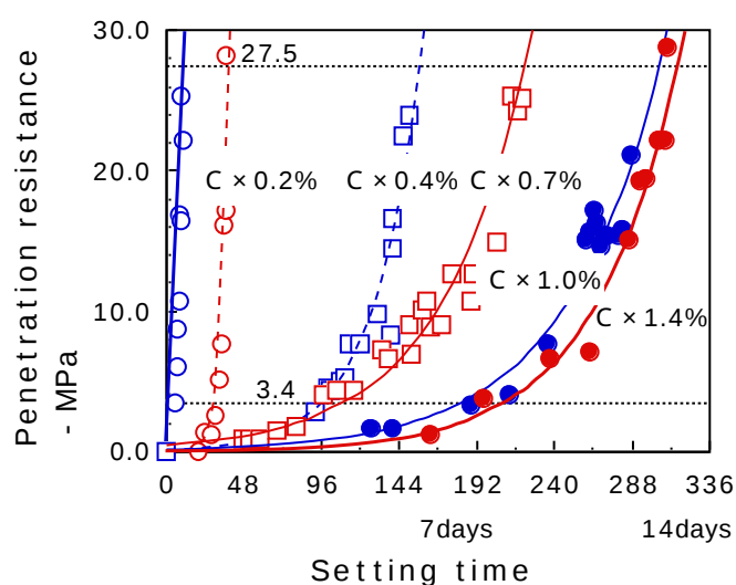
図4 炭酸銅による凝結遅延効果
