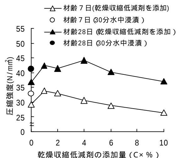
図.3 乾燥収縮低減剤の添加量と圧縮強度の関係
