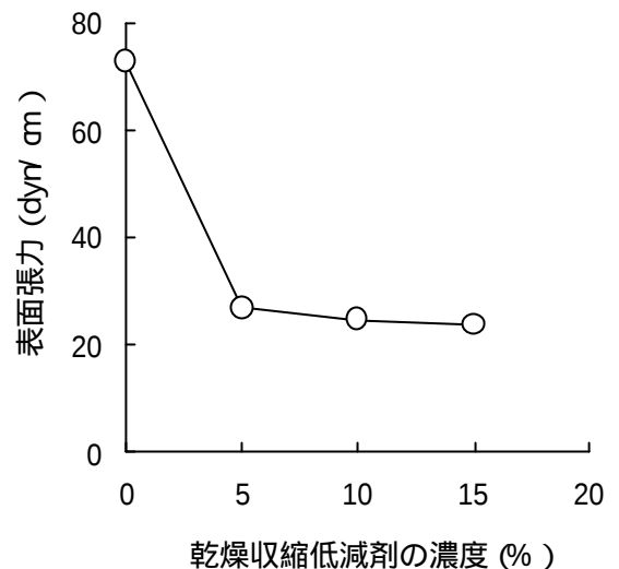
図.1 練混ぜ水中の乾燥収縮低減剤の濃度と表面張力の関係
