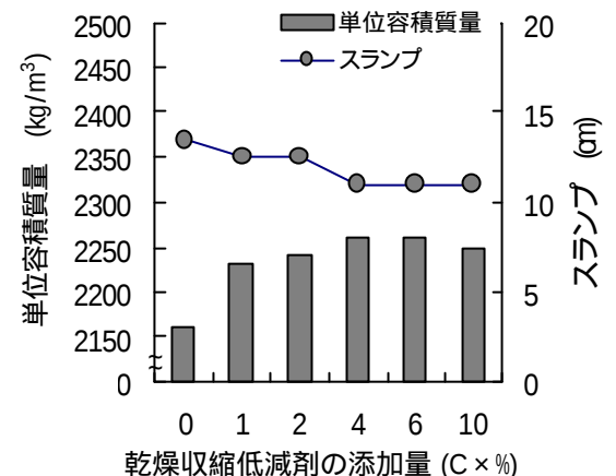
図.2 乾燥収縮低減剤の添加量と再生骨材コンクリートの単位容積質量およびスランプの関係
