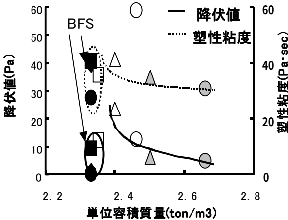
図-2 単位容積質量と降伏値、塑性粘度との関係
