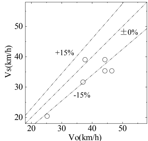
図5 V_o と V_s の比較
