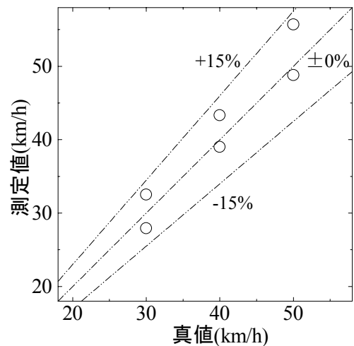
図6 超音波式車両感知器による速度測定誤差
