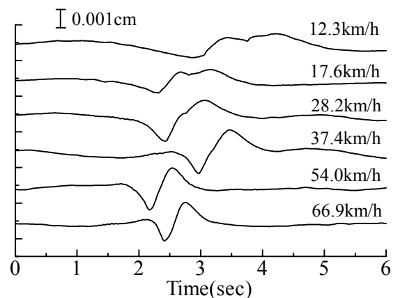
図2 サンプル波形と走行速度
