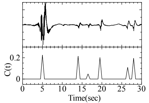
図4 測定結果(上)及び解析結果(下)
