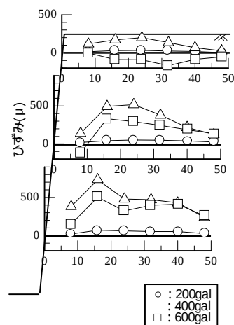
図-8 ひずみ分布(ケース4)
