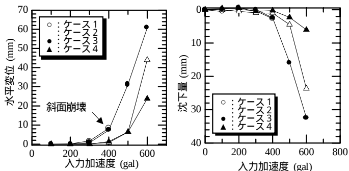
図-3 入力加速度と水平変位
