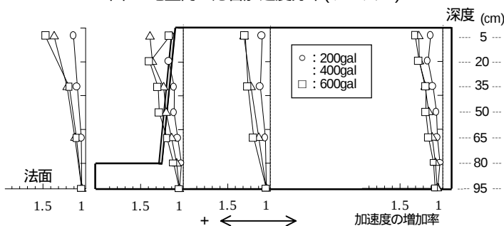
図-6 地盤内の応答加速度分布(ケース4)
