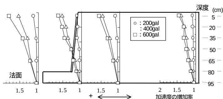
図-5 地盤内の応答加速度分布(ケース2)
