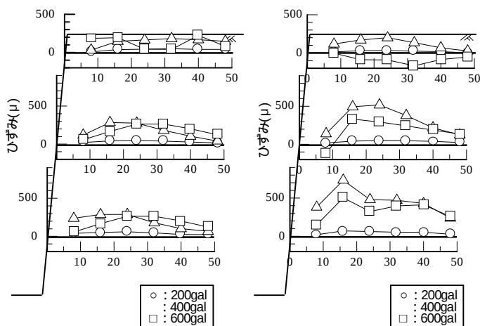
図-7 ひずみ分布(ケース2)
