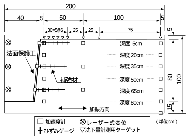
図-1 模型斜面形状およびセンサーの配置図
