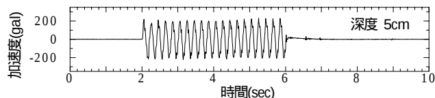
図-2 法面における応答加速度波形（ケース2・200gal）
