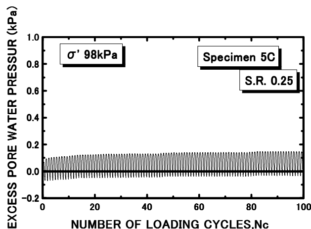
図-2 間隙水圧の発生状況
