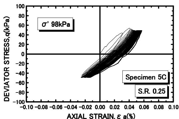
図-1 応力-ひずみ関係
