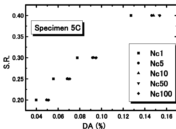
図-3 繰返し応力比とひずみの関係
