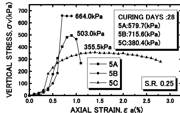
図-5 一軸圧縮試験結果の比較
