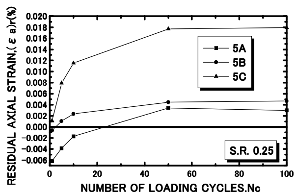
図-4 繰返し載荷回数と残留ひずみの関係
