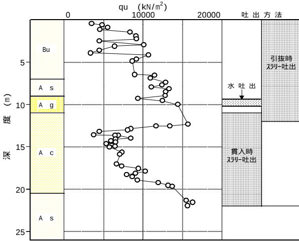
図 - 4 一軸圧縮強さ
