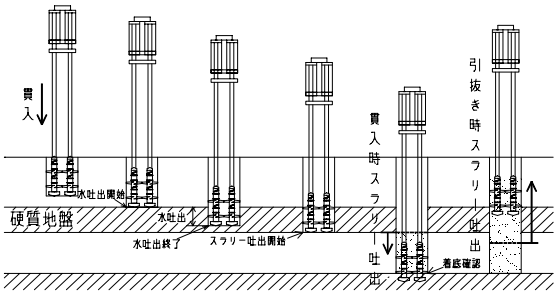
図 - 2 最終施工(1)の施工手順
