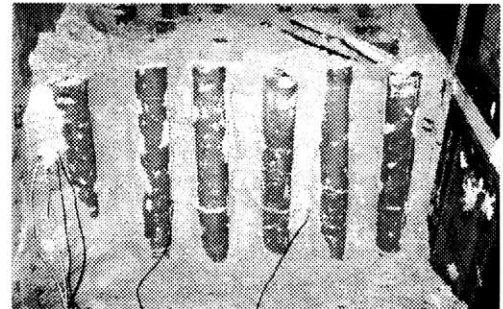
写真1 地盤改良の掘起し状況
