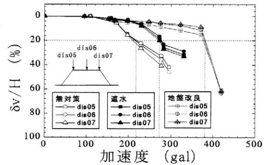
図-3 加振加速度と盛土沈下率の関係
