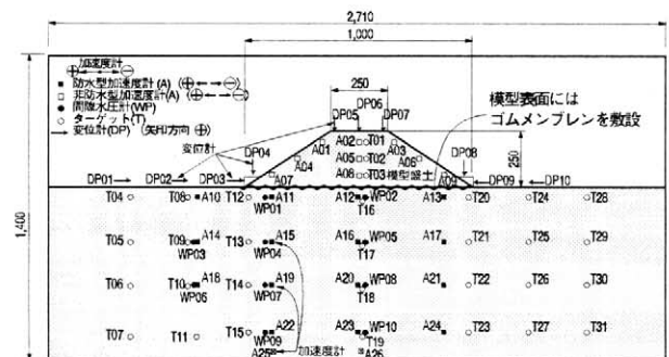
図-1 模型の概要と計測器の配置（底面遮水対策）
