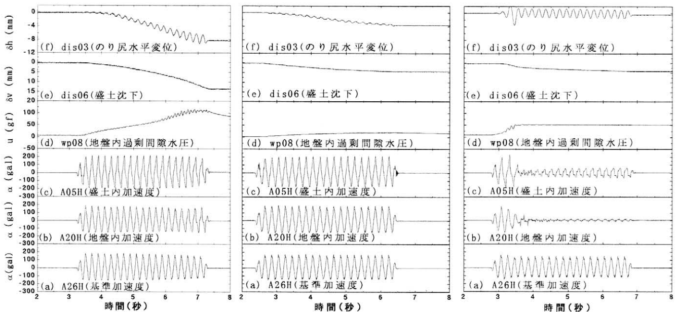
図4 無対策ケース
