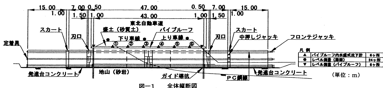
図－1 全体縦断面図
