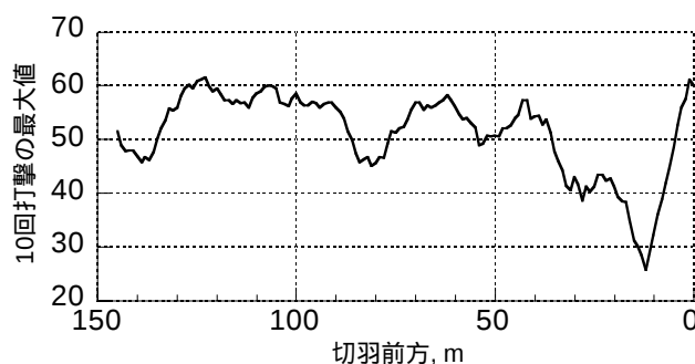
図5 シュミットハンマー反発度
