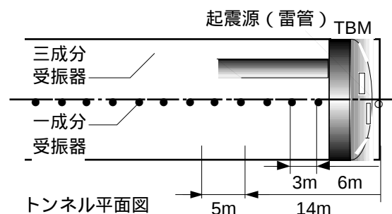
図2 探査の配置
