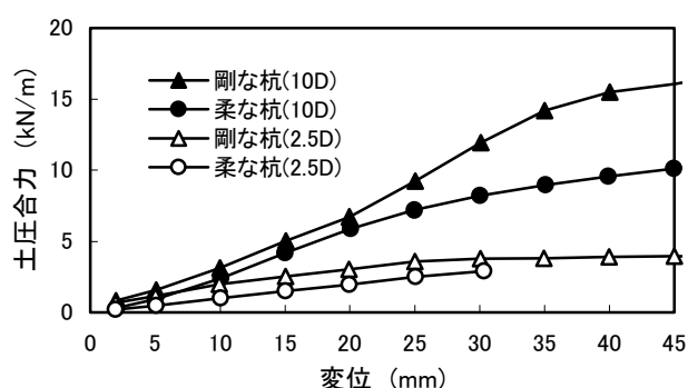
図5 底板変位と土圧合力の関係
