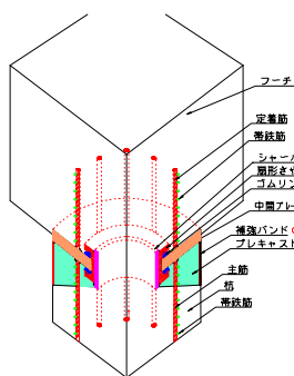
図 - 1 場所打ちジョイント杭構造
