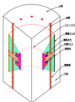
図 - 1 場所打ちジョイント杭構造
