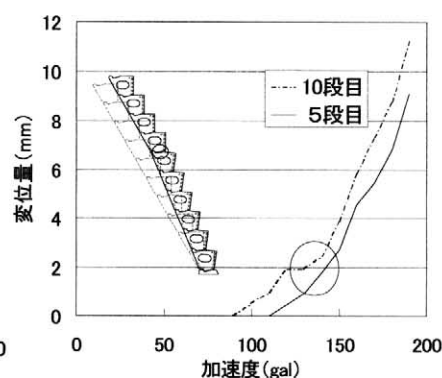
図-5 55°10段における変位の推移
