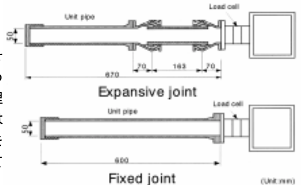
図-2 継手形状
