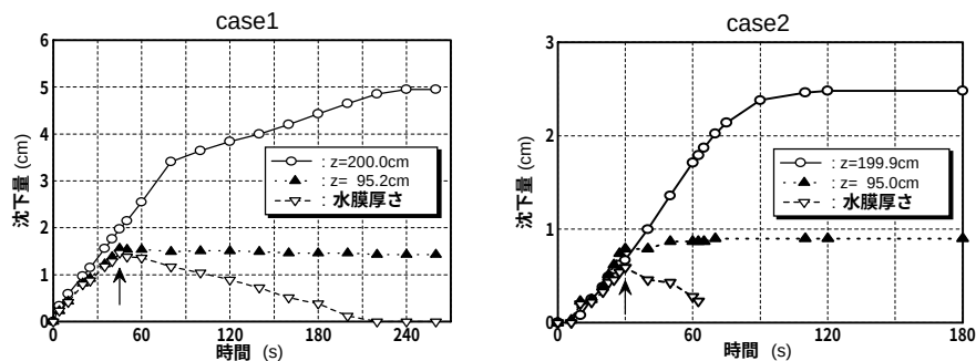
図-4 沈下量及び水膜の厚さ
