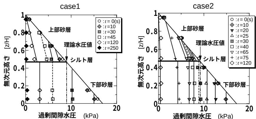
図-3 過剰間隙水圧の時間的变化
