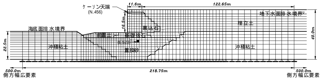
図 2．解析モデル
