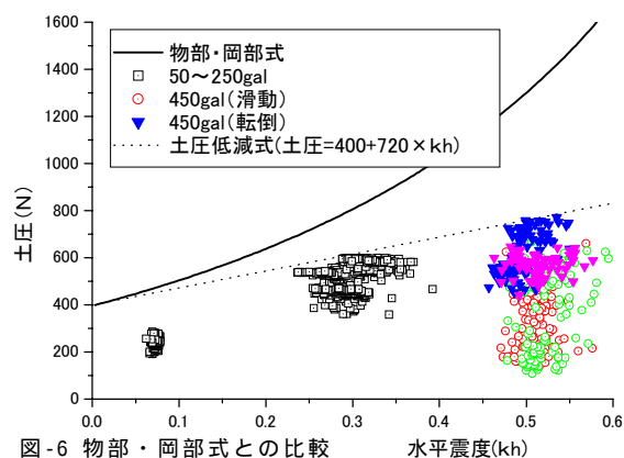
図-6 物部・岡部式との比較
