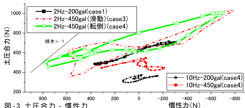
図-3 土圧合力 - 慣性力
