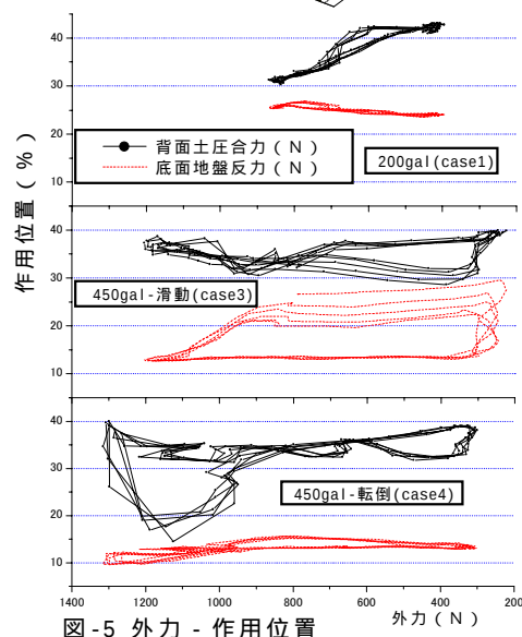
図-5 外力 - 作用位置
