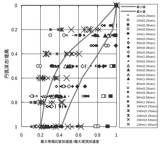
図 - 5 正弦波による結果
