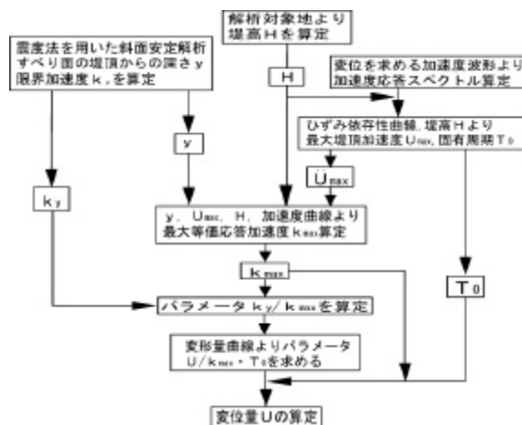
図 - 1 Makdisi & Seed 法の流れ
