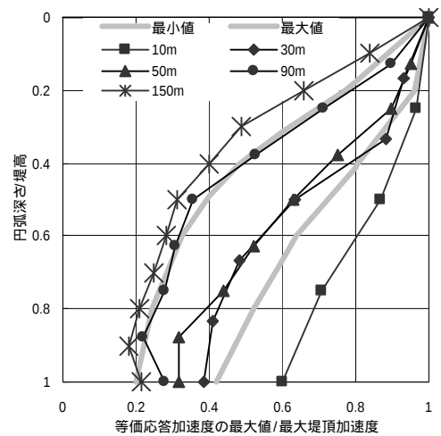
図 - 4 El Centro 波による結果
