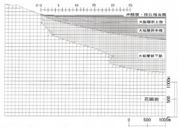
図 - 2 中部地区深層断面モデル
