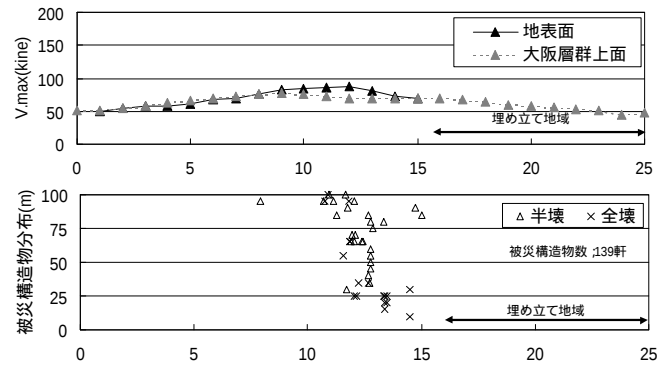
図 - 3 動的応答解析結果(中部地区)
