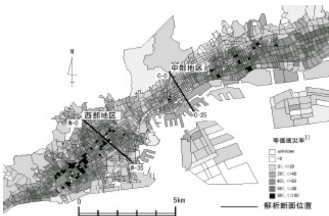
図 - 1 解析断面位置及び被災状況
