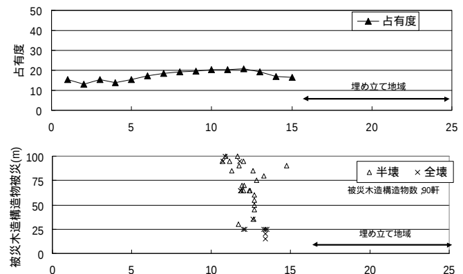
図 - 5 占有度及び木造構造物被害分布(中部地区)
