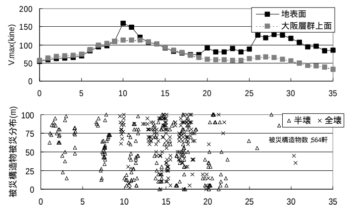
図 - 4 動的応答解析結果(西部地区)
