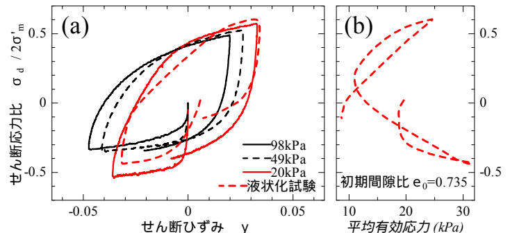
図 - 5 応力～ひずみ関係(TK30 case2)
