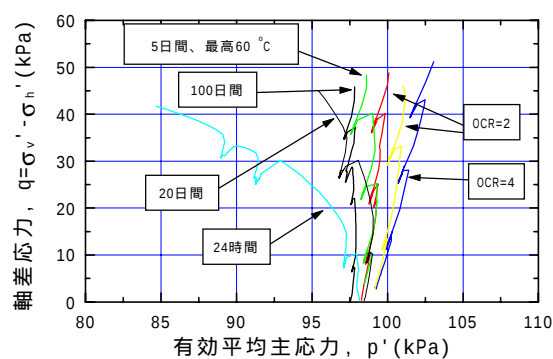
図 4 有効応力経路の比較
