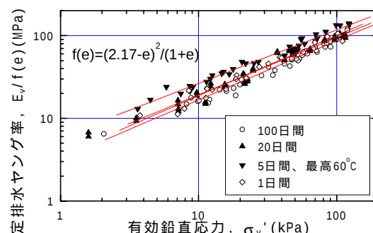
図 3 (a) せん断中の推定排水ヤング率 (1)
