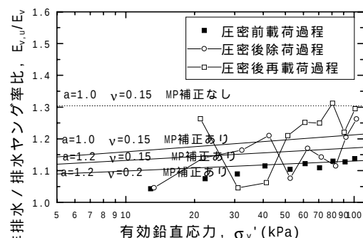
図 2 (d) 過圧密 (OCR=4) 前後でのヤング率比の変化
