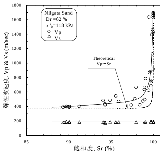
図-2 弾性波速度と飽和度の関係
