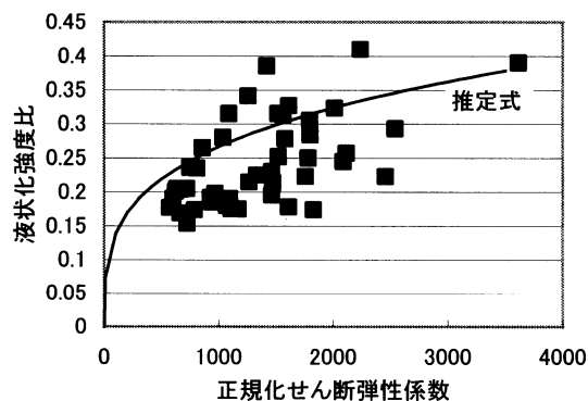
図3 液状化強度比と正規化したせん断弾性数の関係
