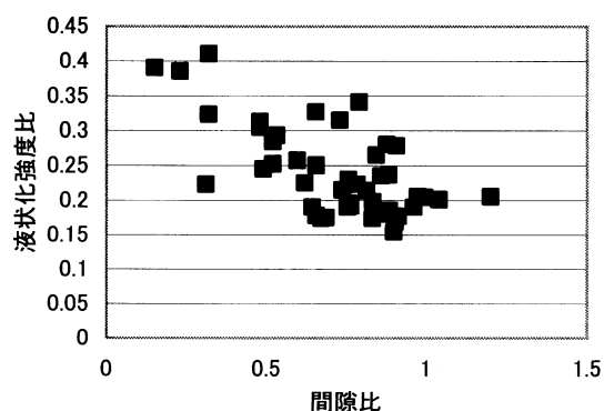
図 1 液状化強度比と間隙比の関係
