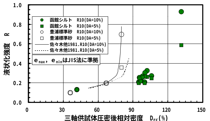
図-1 JIS 法に準拠し求めた相対密度と液状化強度の関係
