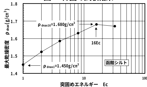
図-3 突固めエネルギーと最大乾燥密度の関係
