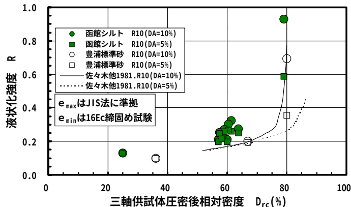
図-5 \rho_{dmax16} を使用して求めた相対密度と液状化強度の関係
