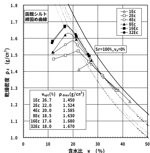
図-2 締固め試験結果
