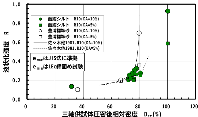
図-4 \rho_{dmax1} を使用して求めた相対密度と液状化強度の関係
