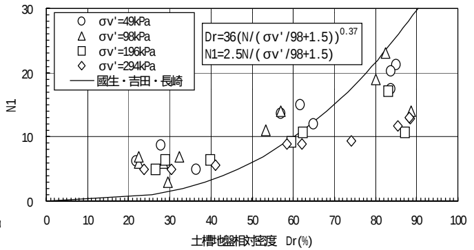
図-4 土槽地盤の相対密度と換算 N 値の関係
