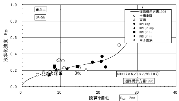
図-6 換算 N 値 N1 と液状化強度の関係 (道路橋示方書 1996)
