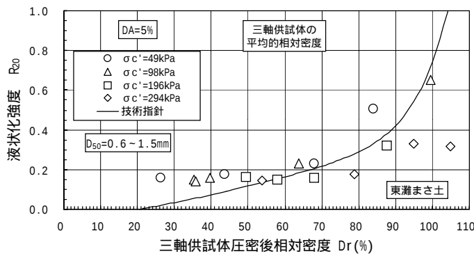
図-3 三軸供試体圧密後の相対密度と液状化強度の関係
