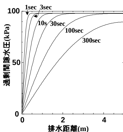
図-7 一次元排水状態における過剰間隙水圧の分布
