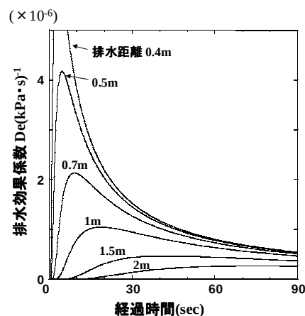
図-8 経過時間・排水距離と De の関係
