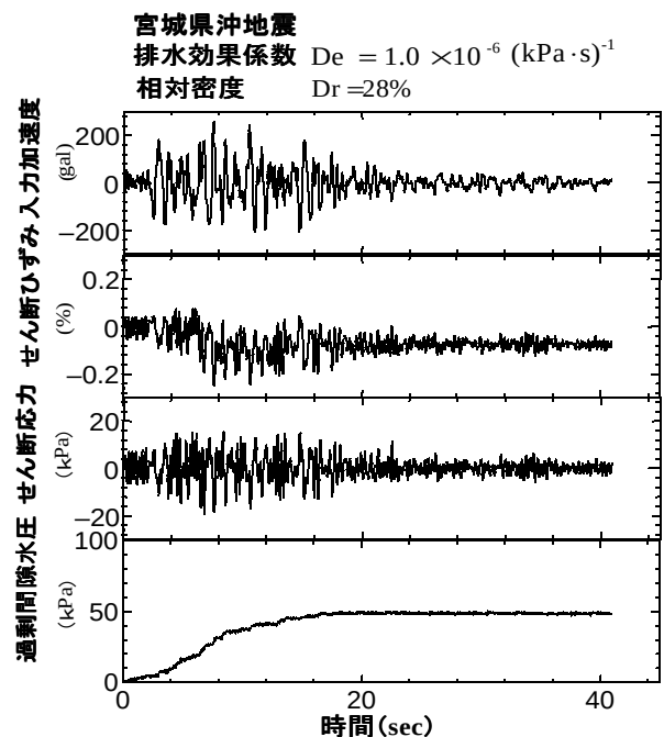
図-1 時刻歴
