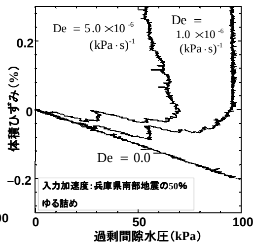
図-5 過剰間隙水圧—体積ひずみ関係
