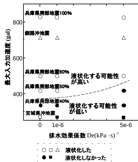
図-6 液状化の可能性と De ・加速度の関係
