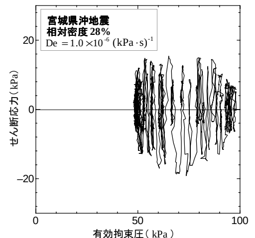
図-3 応力経路
