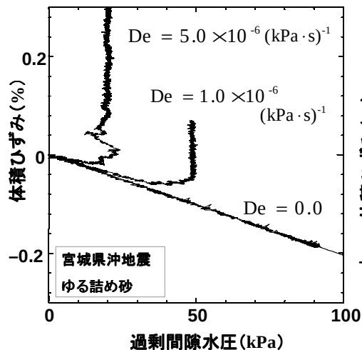
図-4 過剰間隙水圧—体積ひずみ関係
