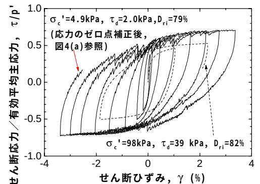
図6 有効応力比とせん断ひずみの関係
