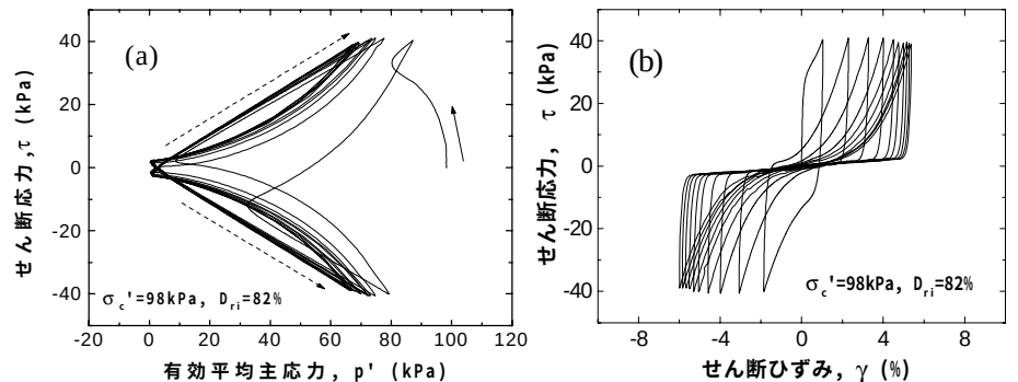
図5 拘束圧98kPaの場合の有効応力経路と応力ひずみ関係
