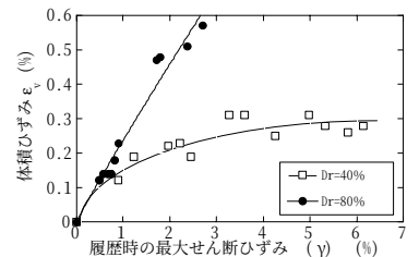
図-9 最大せん断ひずみと体積ひずみの関係
