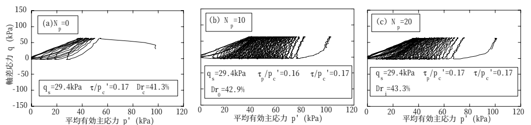
図-2 有効応力経路図 ( Dr=40\% ) (a) N_p=0 (b) N_p=10 (c) N_p=20
