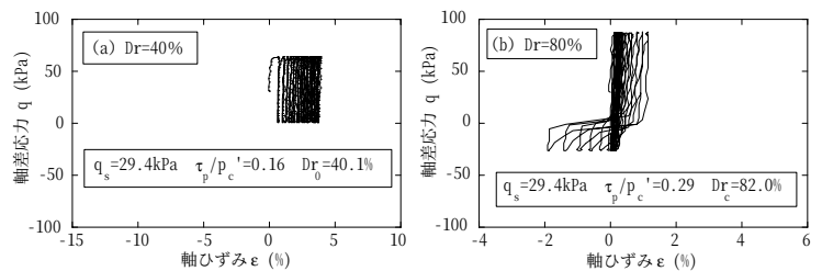
図-4 履歴時の軸ひずみと軸差応力の関係 (a) Dr=40% (b) Dr=80%
