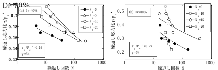
図-5 液状化強度曲線 (a) Dr=40% (b) Dr=80%
