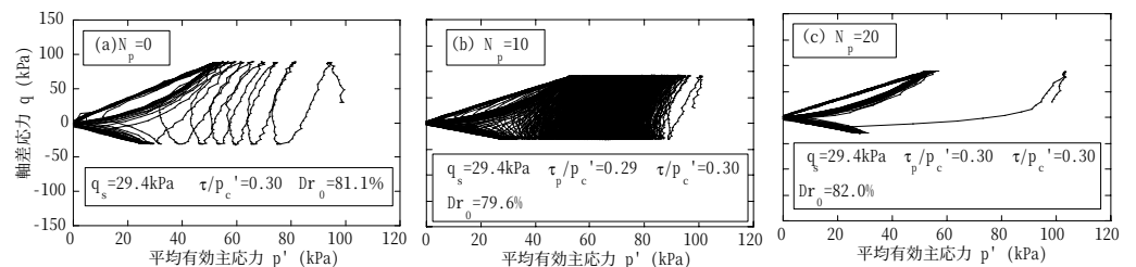
図-3 有効応力経路図 ( Dr=80\% ) (a) N_p=0 (b) N_p=10 (c) N_p=20
