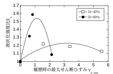
図-6 最大せん断ひずみと液状化強度比の関係
