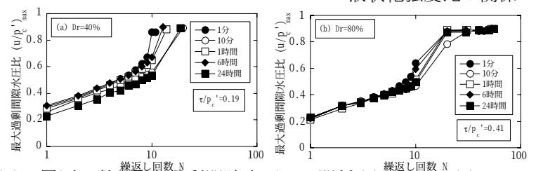
図-7 履歴回数と最大過剰間隙水圧比の関係 (a) Dr=40% (b) Dr=80%
