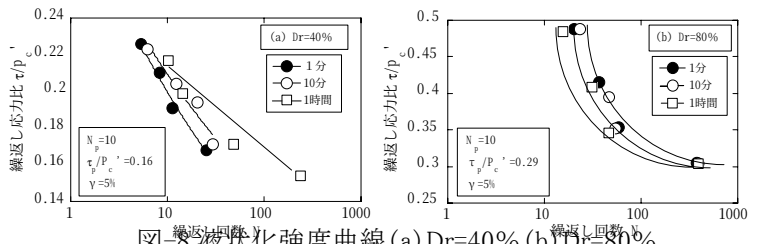
図-8 液状化強度曲線 (a) Dr=40% (b) Dr=80%
