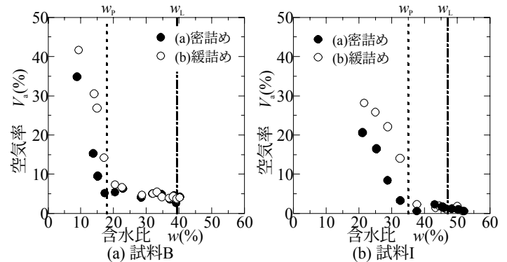
図-4 空気率と含水比の関係
