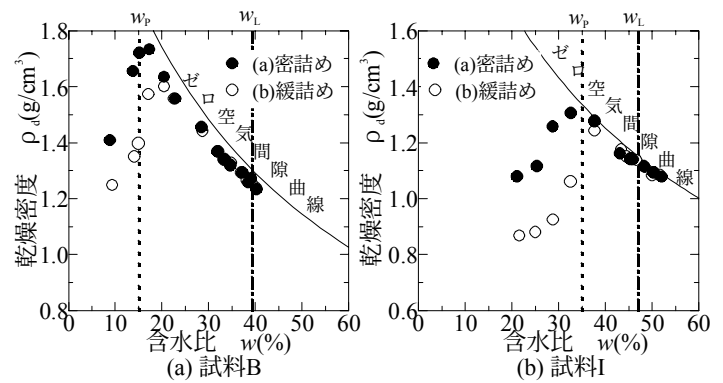
図-2 乾燥密度と含水比の関係
