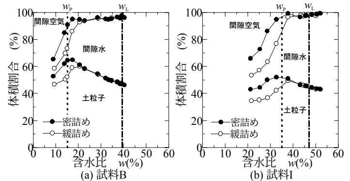
図-3 体積割合と含水比の関係
