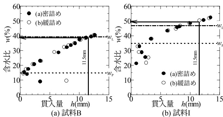
図-1 含水比と貫入量の関係
