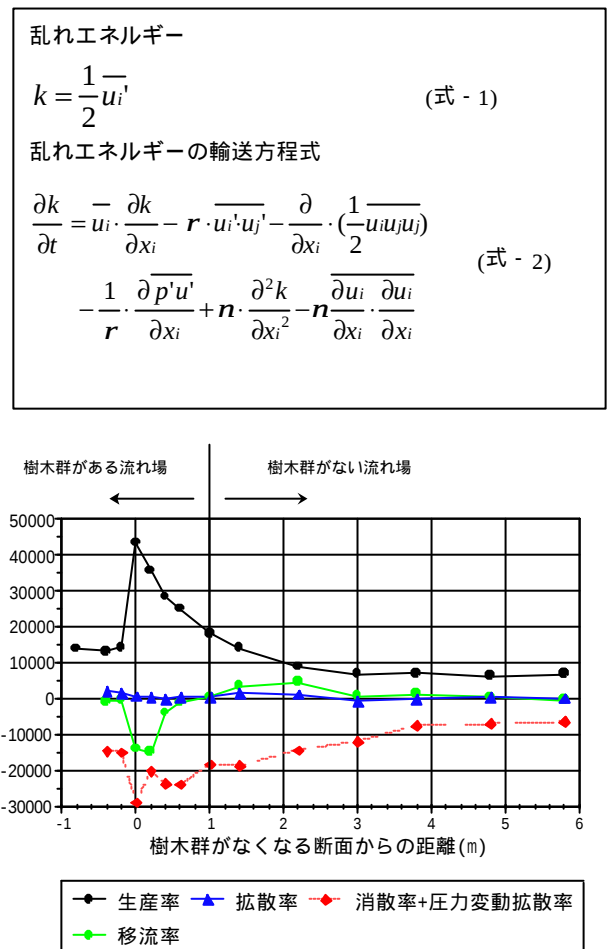
図-4 乱れエネルギーの収支の縦断変化
