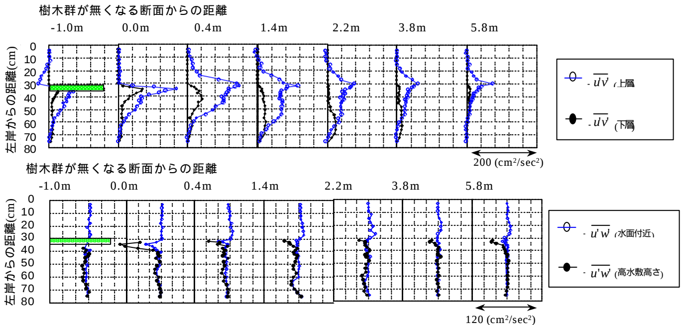
図 - 3 Reynolds 応力 ( -\overline{u'v'} , -\overline{u'w'} ) の縦断变化
