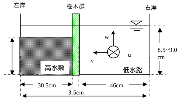
図 - 1 水路断面図
