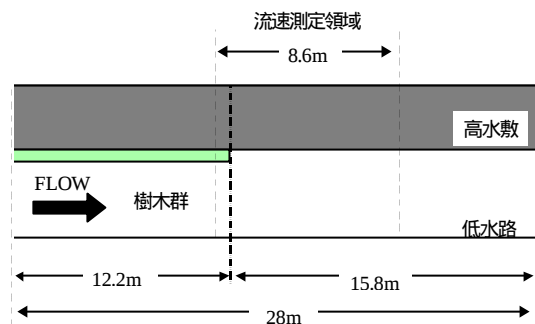
図 - 2 水路平面図
