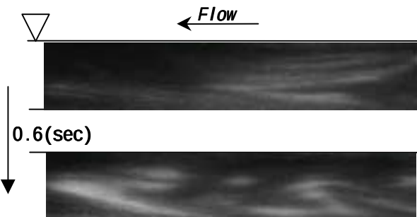
写真-3 CaseB1(植生境界部)
