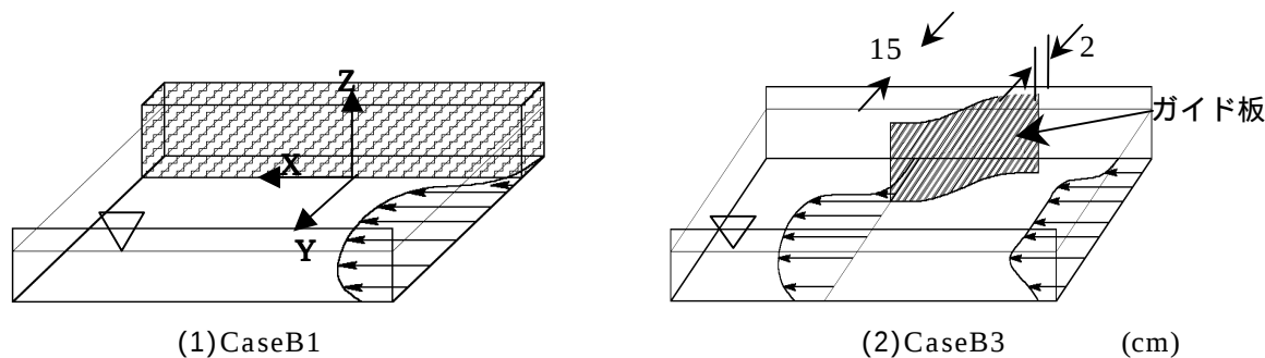
図-1 実験ケースの模式図
