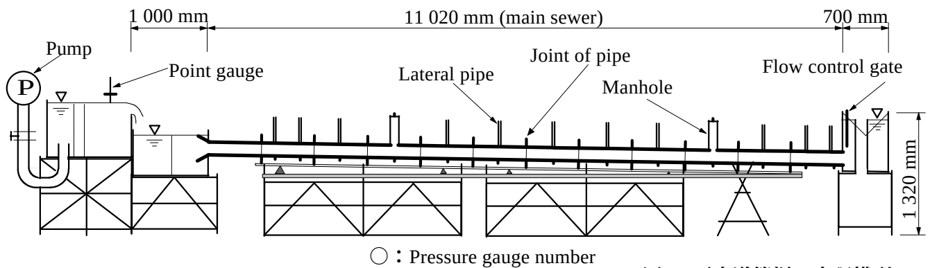
図-2 下水道管渠の水理模型
