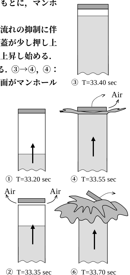
図-6 マンホール蓋飛散のメカニズム
