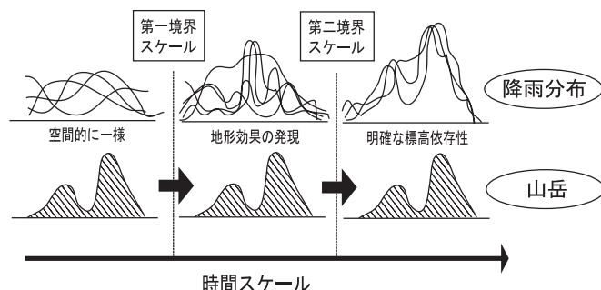
図1：時間スケール階層構造の概念図
