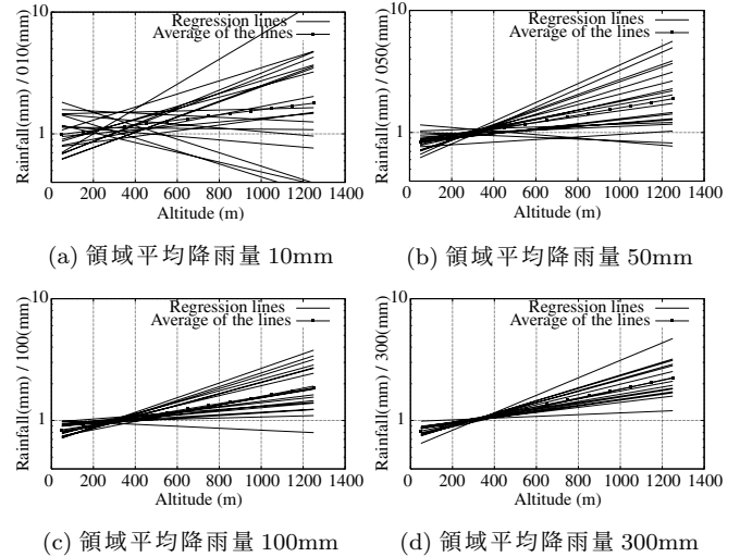
図4：各積分降雨量における標高層別化回帰直線
