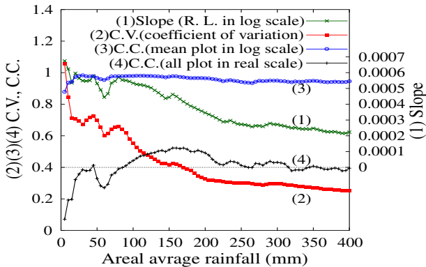
図3：領域平均積分降雨量に対する分布特性の変化（積算期間98/09/01 - 98/10/17）
