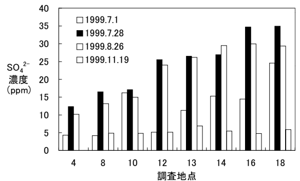
図 - 3 各地点での硫酸イオン濃度
