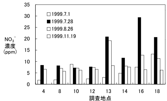
図 - 2 各地点での硝酸イオン濃度
